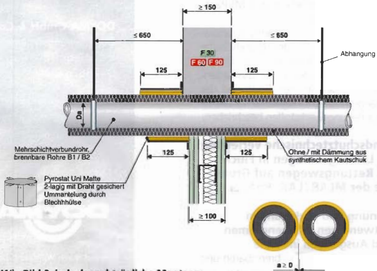
Bild 4 · Wie Bild 3, jedoch nachträgliche Montage.
