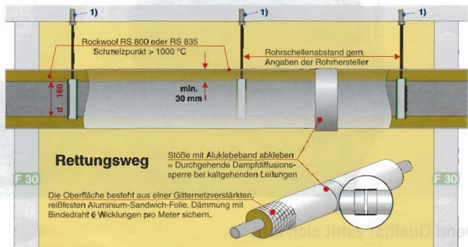
Bild 1 · Brennbare Rohre mit durchgehender Ummantelung aus nichtbrennbaren Dämmstoffen, Dicke min. 30 mm (die Ausführung entspricht der Gutachterlichen Stellungnahme Nr. 3335 / 1111-Mer der MPA Braunschweig. Download unter www.MLPartner.de > Download > Herstellerdokumente > Rockwool Verlegung in Rettungswegen Bild S. 29).
