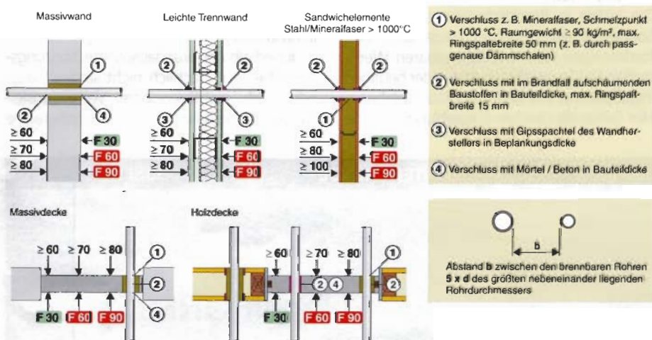
Bild 7 - Abschottung von Einzelrohren nach den Erleichterungen der MLAR/LAR/RbALei bis d \leq 32 mm.
