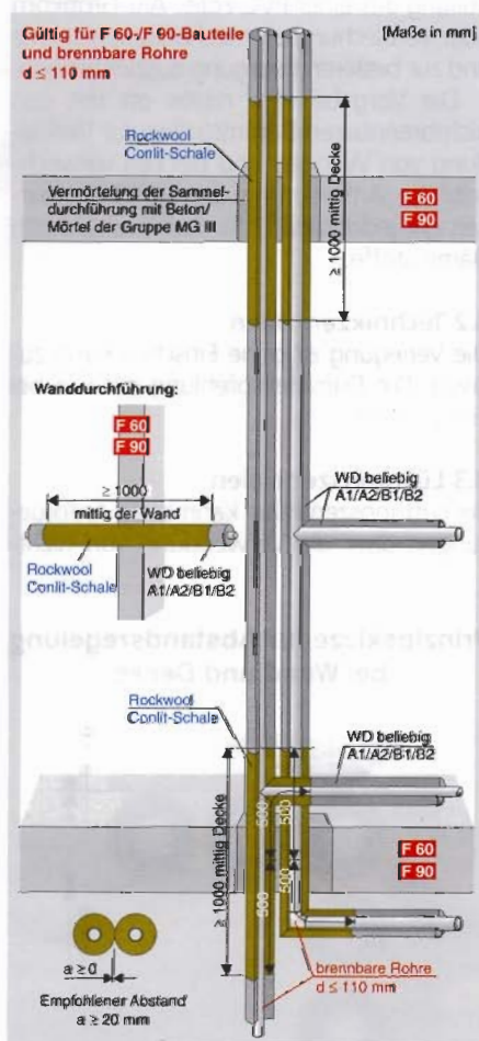
Bild 2 · R 30 bis R 90-Rohrabschottungen für brennbare Rohre – gilt für Wände und Decken (Verwendungsnachweis nach Rockwool ABP P-3726/4140-MPA BS).
