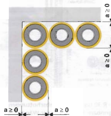
Bild 5 · Abstandsregelung zu Bild 3 und 4.
