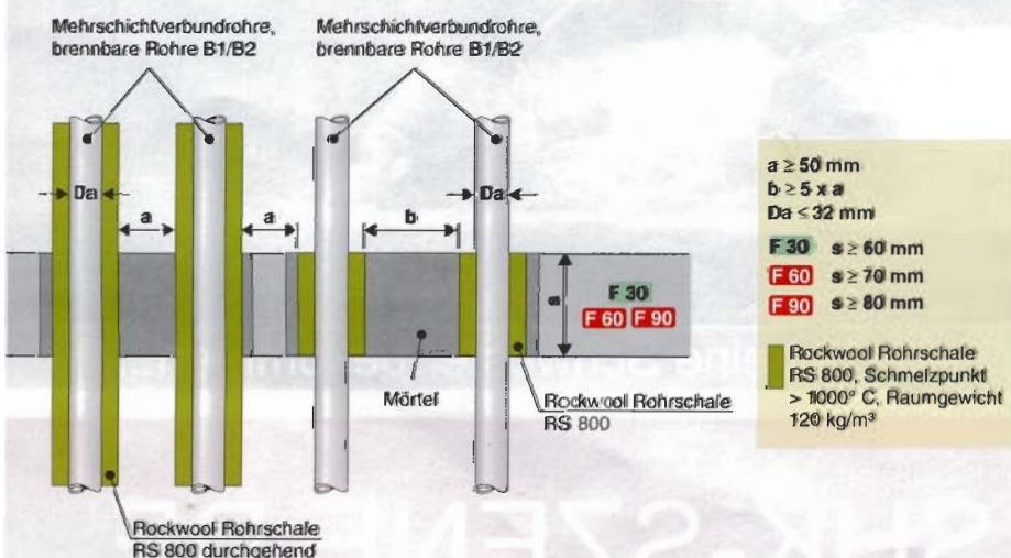
Bild 8 - Leitungsdurchführungen brennbar d \leq 32 mm mit der Rockwool Rohrschale RS 800, Dämmdicke 20-30 mm.
