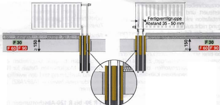
Bild 6 · Heizkörperanschlussleitung mit brennbaren Versorgungsrohren mit einer Dämmung aus synth. Kautschuk (50 % nach EnEV) + Pyrostat UNI unter Berücksichtigung der engen Anschlussabstände von Fertigventilgruppen.
