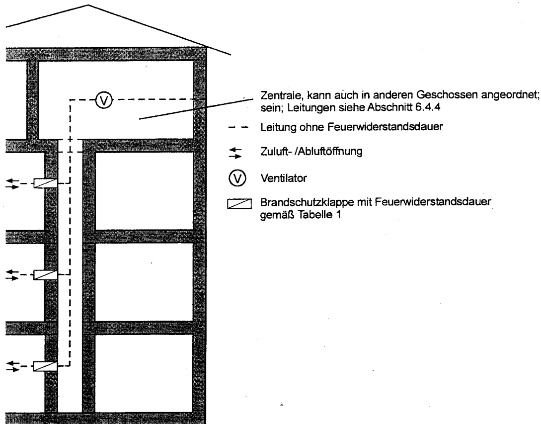
Bild 1.2: Schachtlösung
