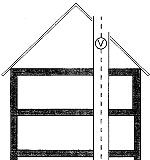
Bild 2.2 Schachtlösung
