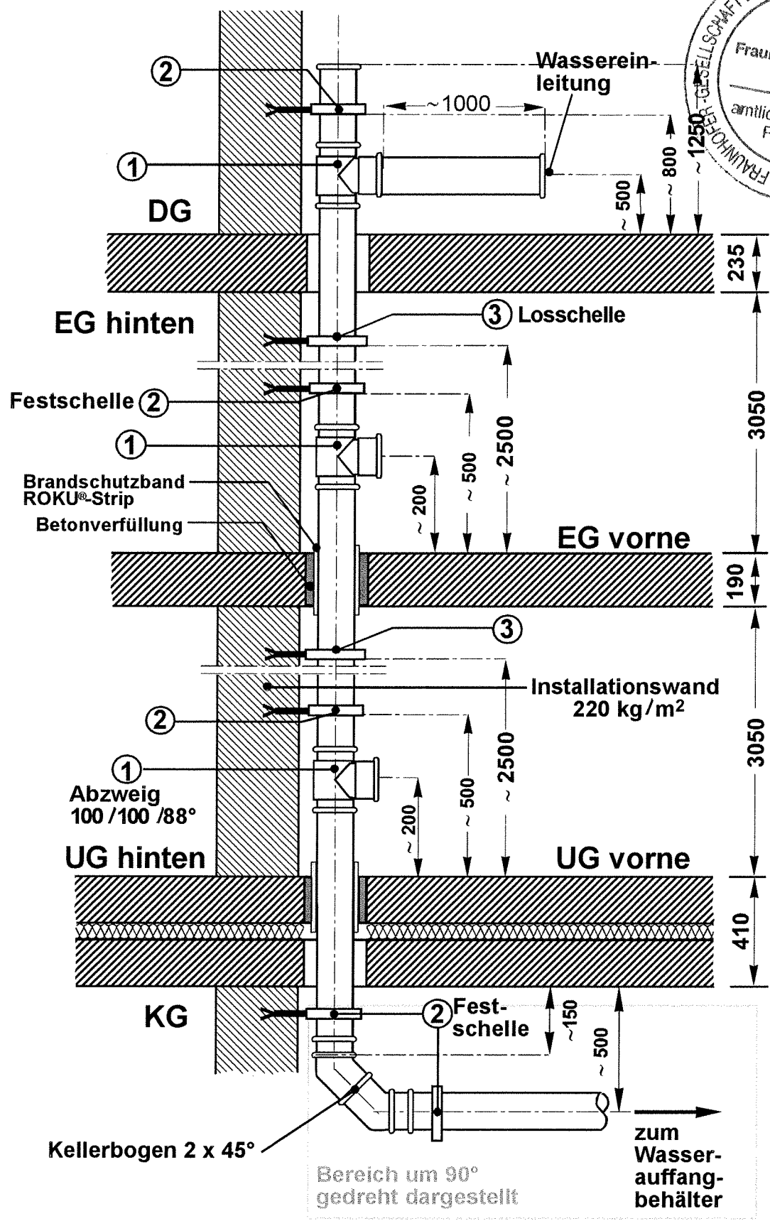
Bild 3 Fa. Rolf Kuhn. Installationsplan für alle Versuchsaufbauten. Die Rohrschellen waren bei allen Messungen an derselben Stelle angebracht. Bei den Messungen wurde das Brandschutzband "ROKU®-Strip" bzw. "ROKU®-Strip L 110" bzw. "ROKU®-Strip L 110 mit doppelseitigem Schaumstoffklebeband" in den Deckendurchbrüche EG/UG und UG/KG angebracht. Alle Maße in mm, Darstellung nicht maßstabsgerecht.
